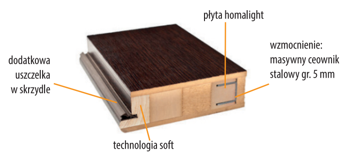
PRZEKRÓJ SKRZYDŁA REDAN
