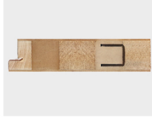
WZMOCNIENIE MASYWNYM CEOWNIKIEM STALOWYM
